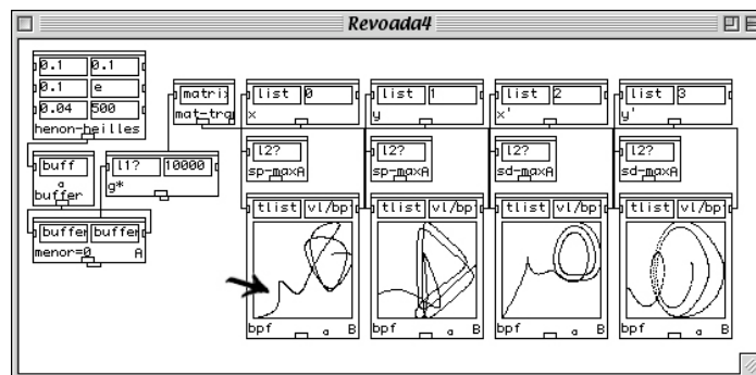
Figura 5. Patch construído no software PatchWork mostrando os gráficos no espaço de fases para as variáveis do sistema de Hénon-Heiles combinadas duas a duas ((x,y) , (x,y') , (x',y) e (x',y') ). Note-se o
